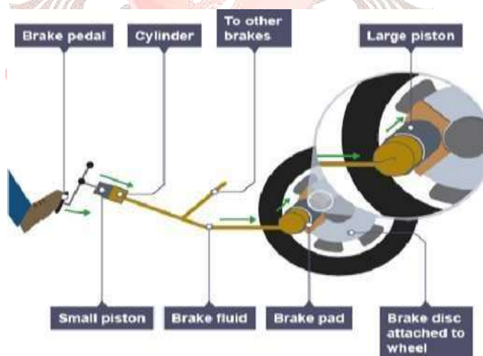
Fig.no. 3: Breaking fundamentals
